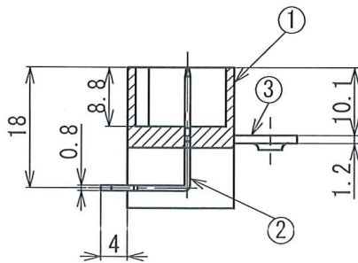
断面図 C-C
