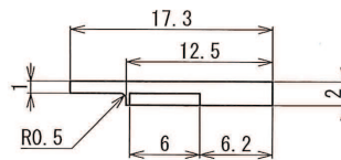
A矢視図 (2/1)
