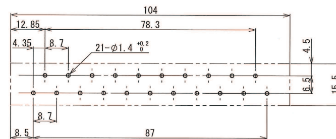
プリント基板寸法
