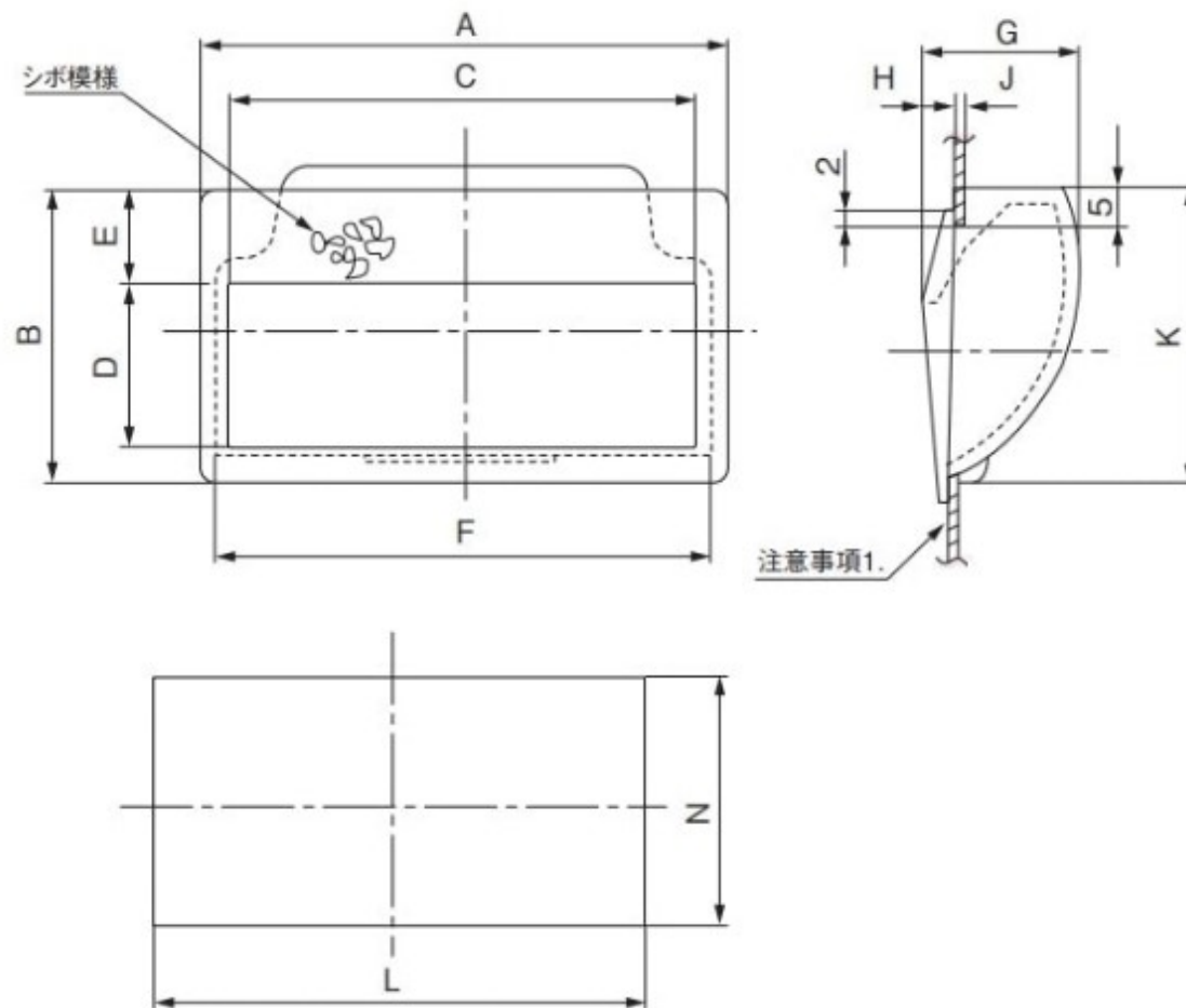
取付穴図
