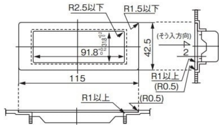
取付穴図
