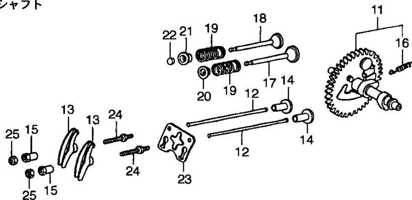
カムシャフト
