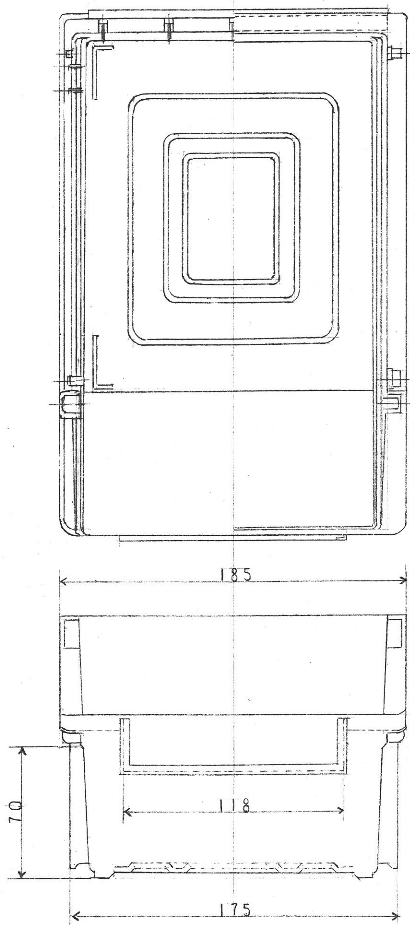
裏面図
