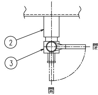
A部詳細
