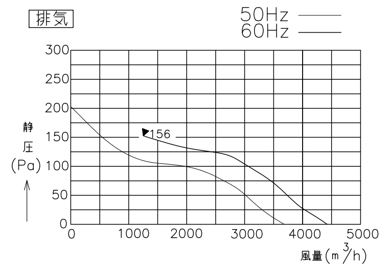
■ 静圧－風量特性
