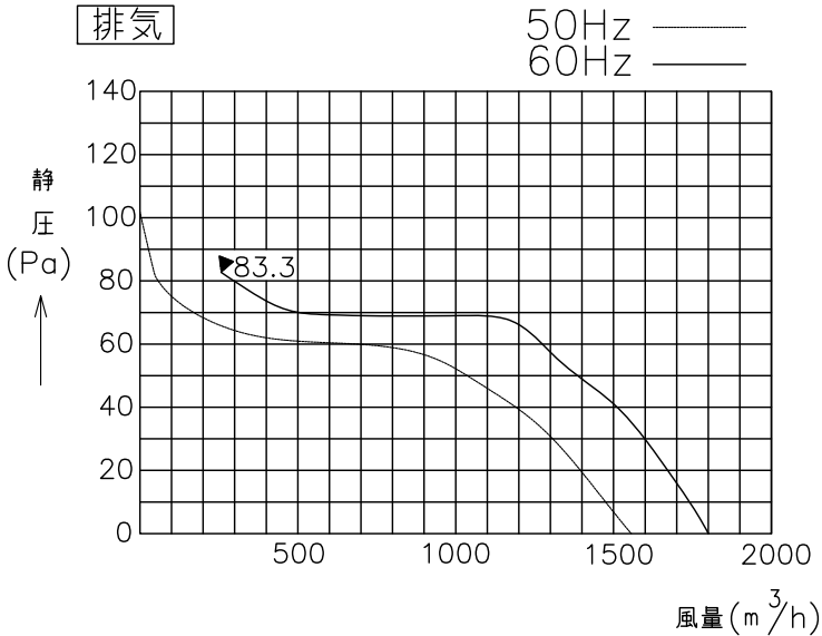
■ 静圧－風量特性
