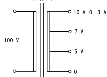
結線図
