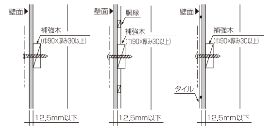
図3 湿式壁
