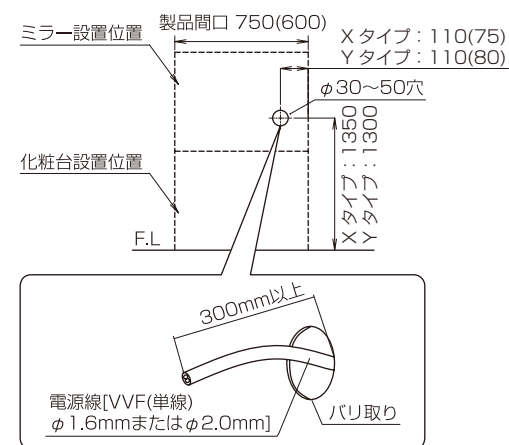
図1 直結配線の穴位置
