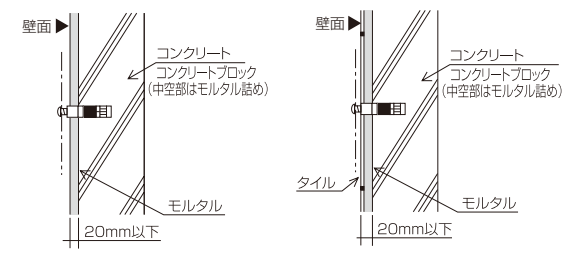
図3 湿式壁
