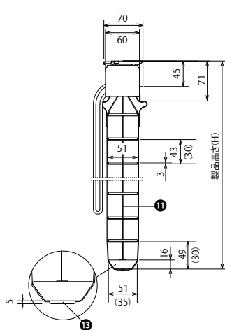
側面図 (mm)
