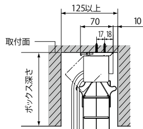
カーテンボックス内 納まり図 (mm)
