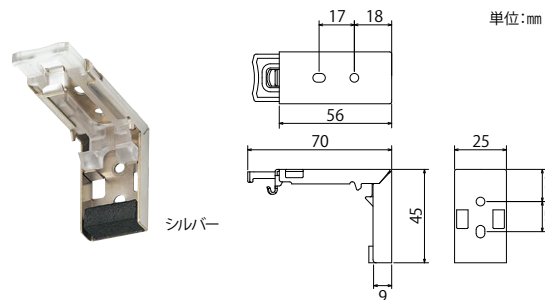
付属品 (ブラケット)
