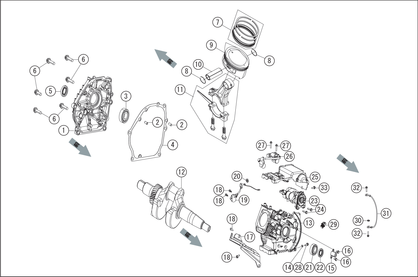
型式名 GV-30IS-AAA-0 (065861701) ケースカバー / ピストン・シャフト / クランクケース・イグニッションコイル * 表示価格は部品一個あたりの単価です
