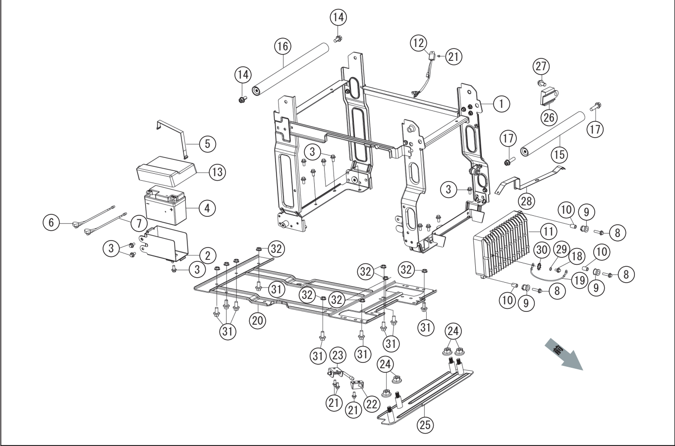
型式名 GV-30IS-AAA-0 (065861701) フレーム・バッテリー・インバーター
