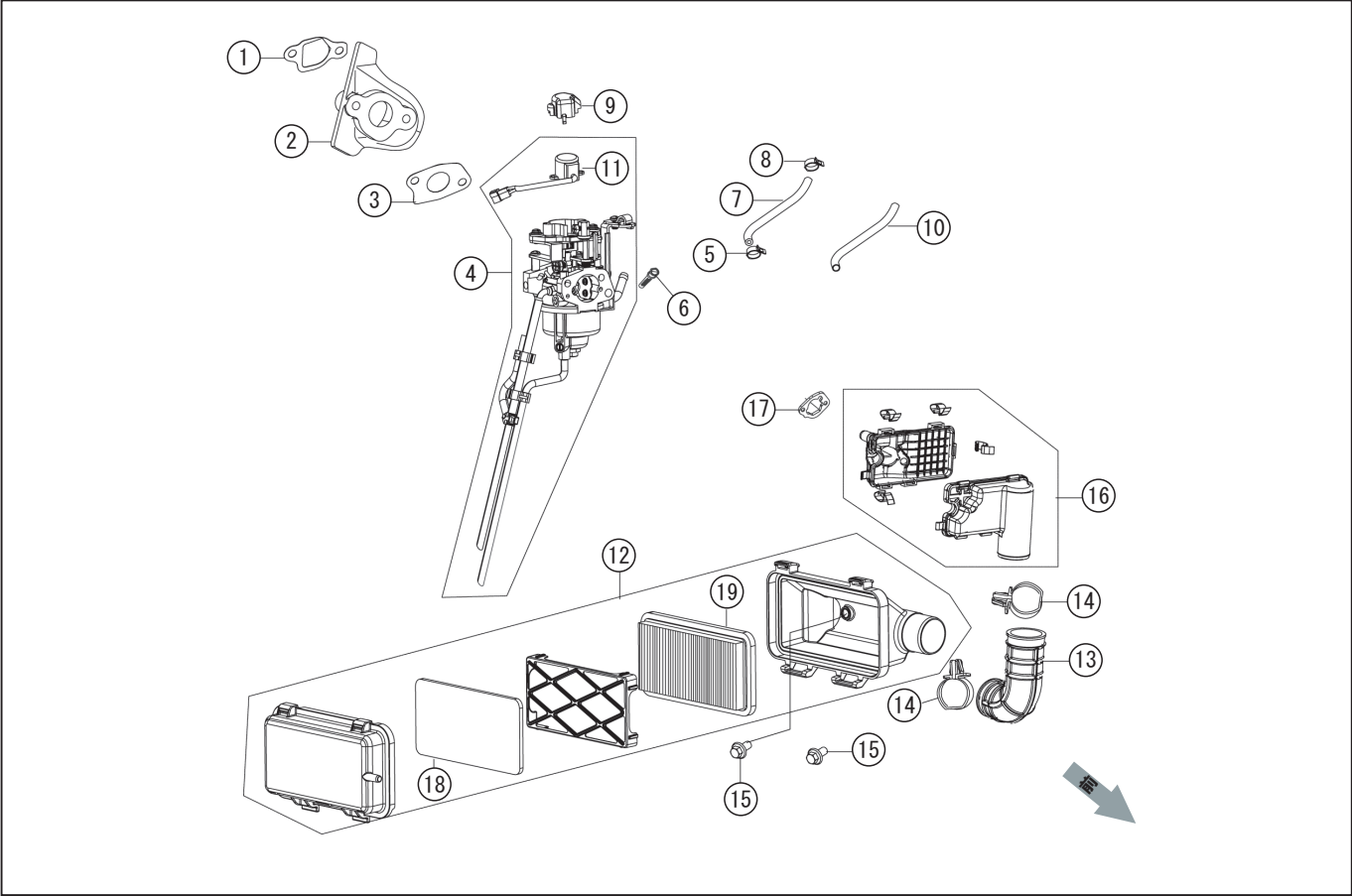
型式名 GV-30IS-AAA-0 (065861701) キャブレーター / エアクリーナー
