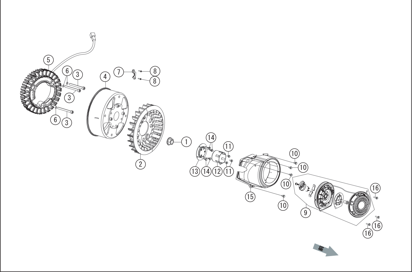
型式名 GV-30IS-AAA-0 (065861701) ローター・ステーター / ファンカバー・リコイルスターター
