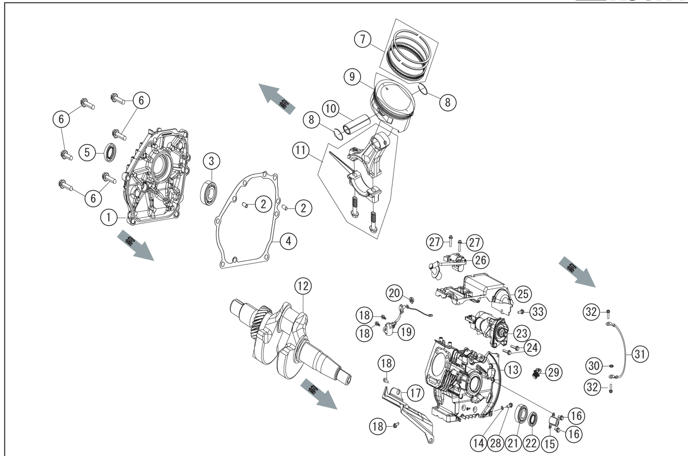
型式名 GV-30IS-AAA-0 (065861701) ケースカバー / ピストン・シャフト / クランクケース・イグニッションコイル
