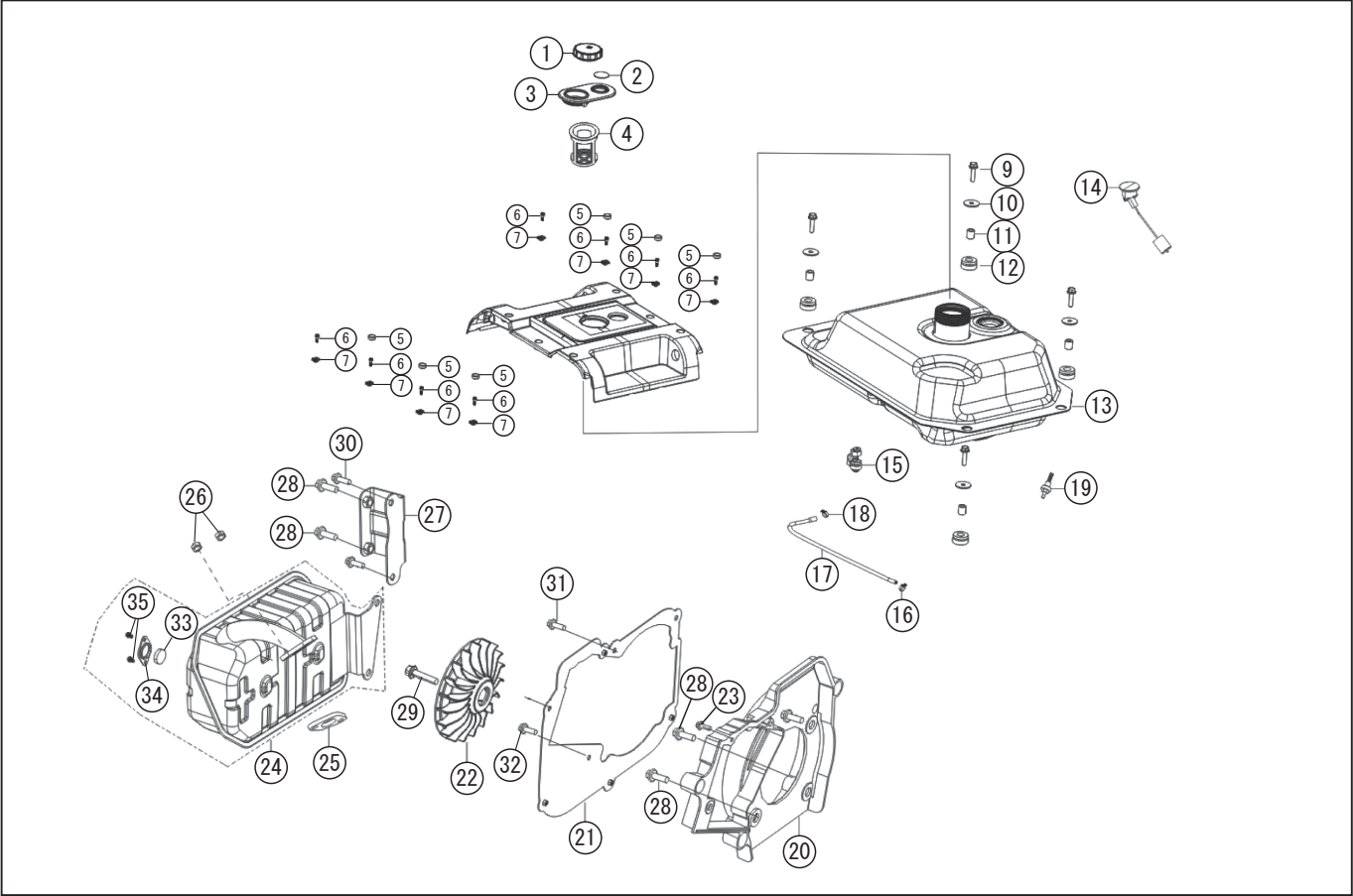
型式名 GV-29I-AAA-0 (065863401) 燃料タンク / マフラー *使用個数は1台に使用している個数です。入り数ではありません *表示価格は部品一個あたりの税抜き単価です
