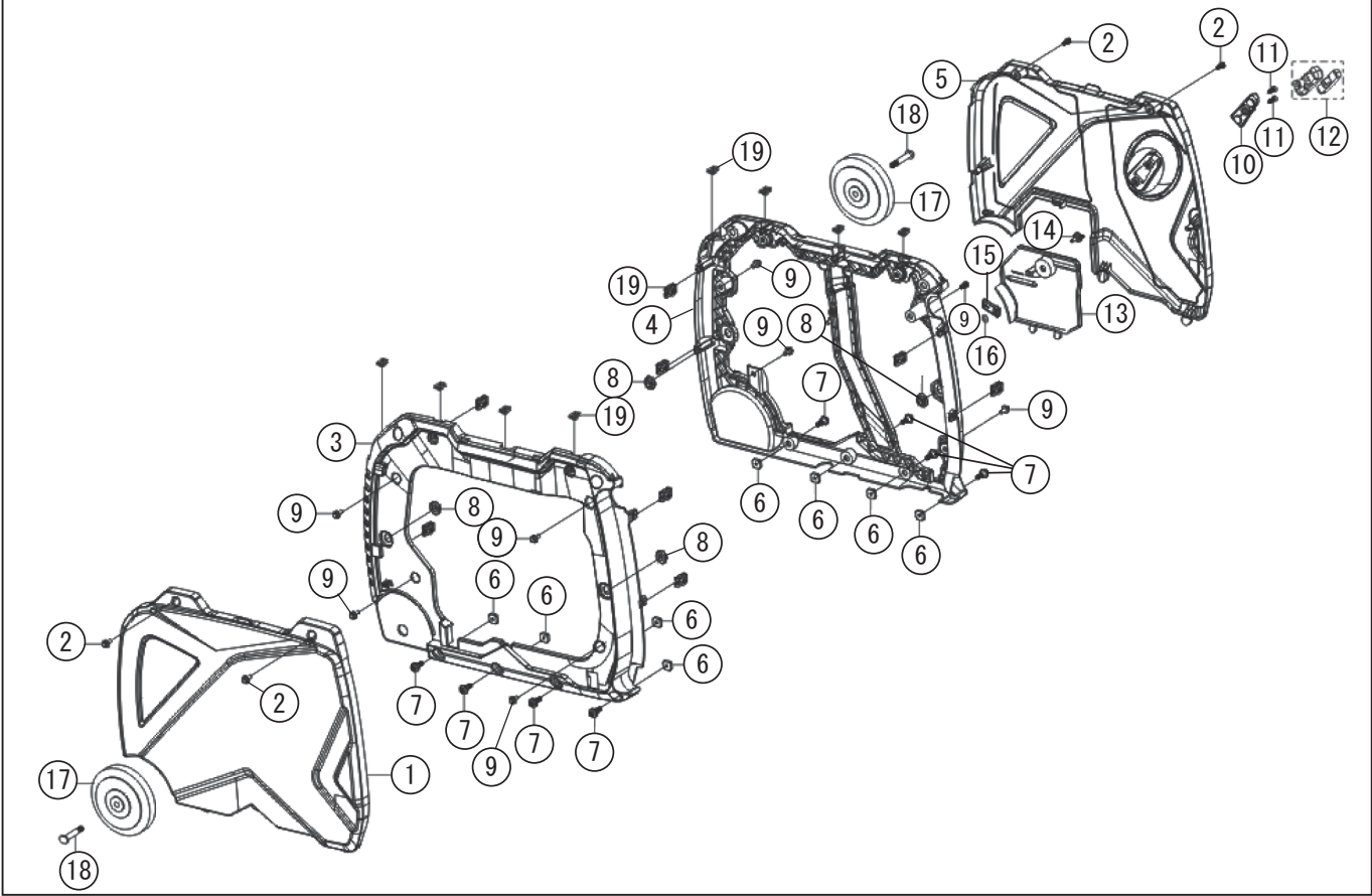
型式名 GV-29I-AAA-0 (065863401) カバー
