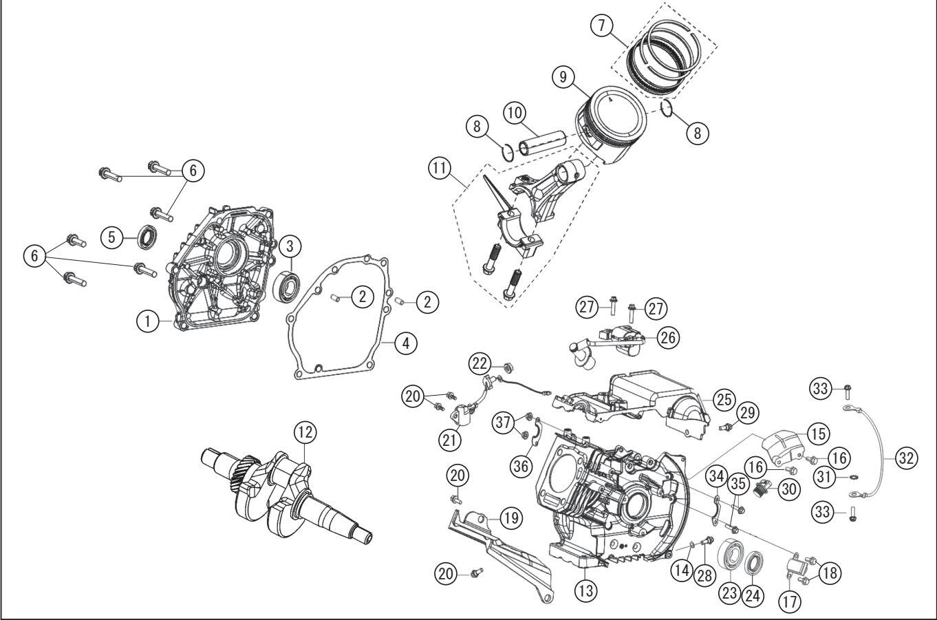
型式名 GV-29i-AAA-0 (065863401) ケースカバー／ピストン、シャフト／クランクケース、イグニッションコイル *使用個数は1台に使用している個数です。入り数ではありません *表示価格は部品一個あたりの税抜き単価です
