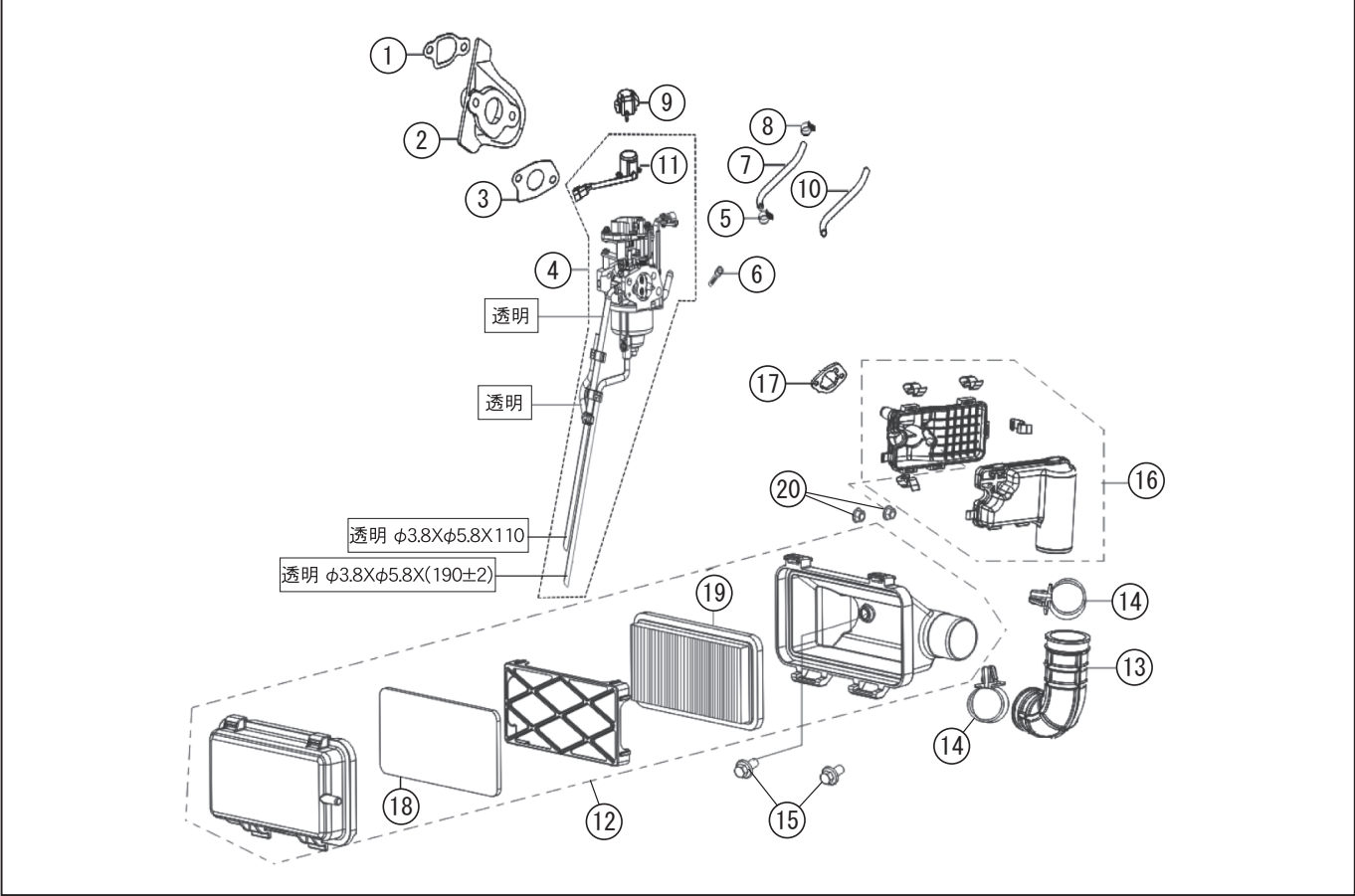
型式名 GV-29I-AAA-0 (065863401) キャブレーター / エアクリーナー *使用個数は1台に使用している個数です。入り数ではありません *表示価格は部品一個あたりの税抜き単価です
