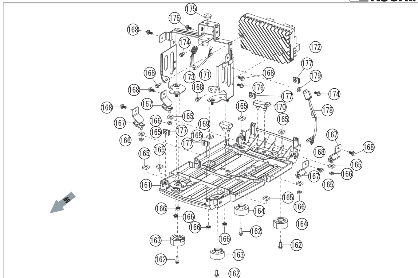
型式名 GV-16I-AAA-4 (065856511) インバーター、底板
