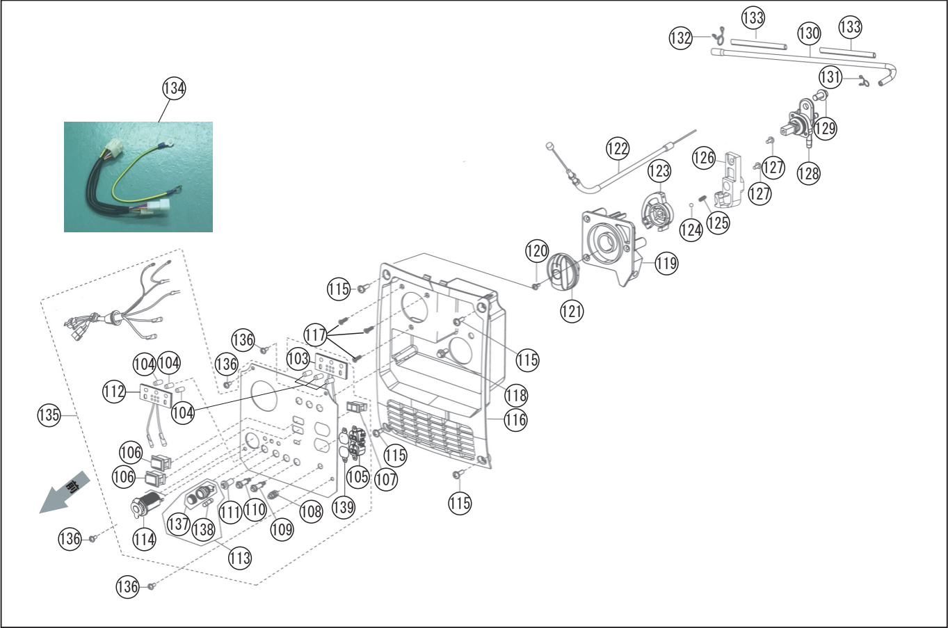
型式名 GV-16I-AAA-4 (065856511) コントロールパネル
