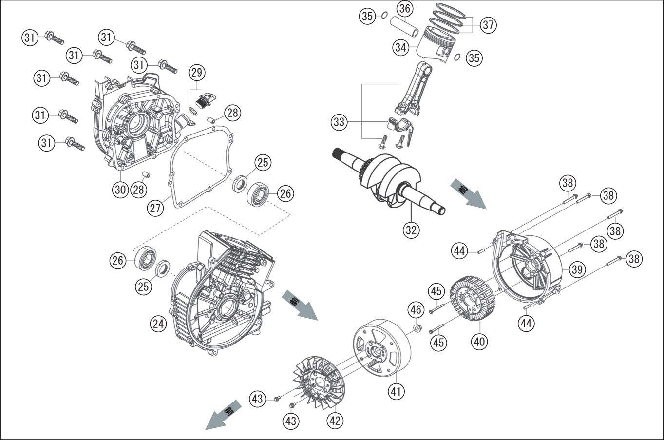
型式名 GV-16I-AAA-4 (065856511) クランクケース、ケースカバー／ピストン、シャフト／ローター、ステーター *使用個数は1台に使用している個数です。入り数ではありません *表示価格は部品一個あたりの税抜き単価です
