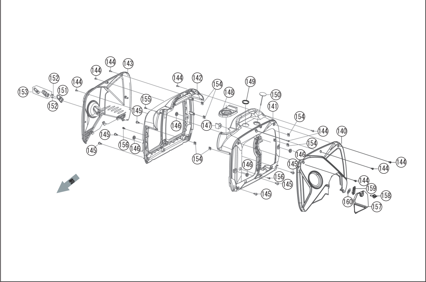
型式名 GV-16I-AAA-4 (065856511) カバー *使用個数は1台に使用している個数です。入り数ではありません *表示価格は部品一個あたりの税抜き単価です
