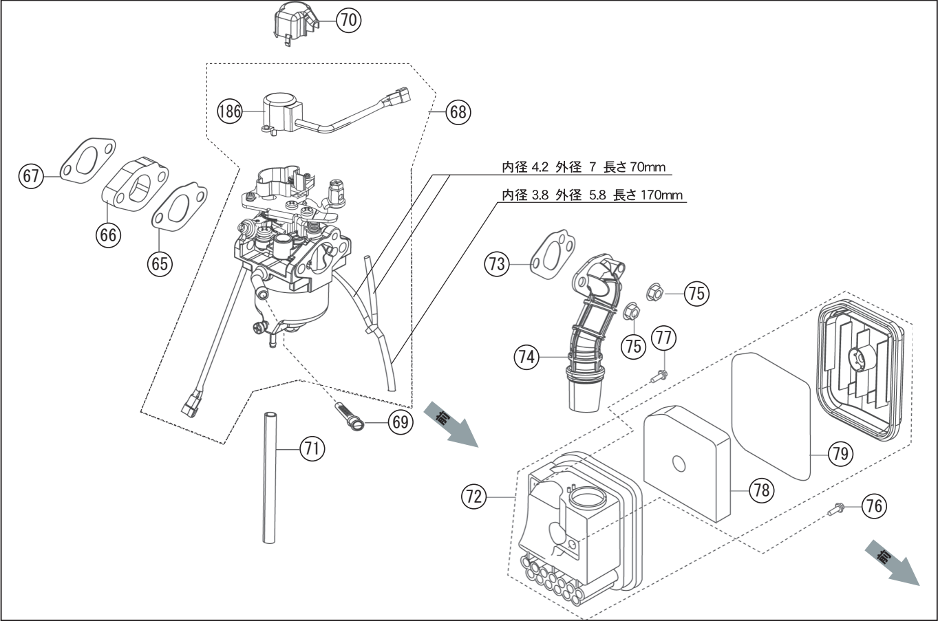
型式名 GV-16I-AAA-4 (065856511) キャブレター / エアクリーナー *使用個数は1台に使用している個数です。入り数ではありません *表示価格は部品一個あたりの税抜き単価です
