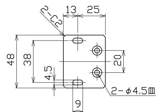
座金詳細図
