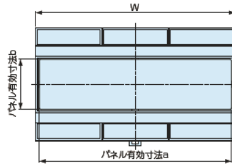
H53-9MG-□
