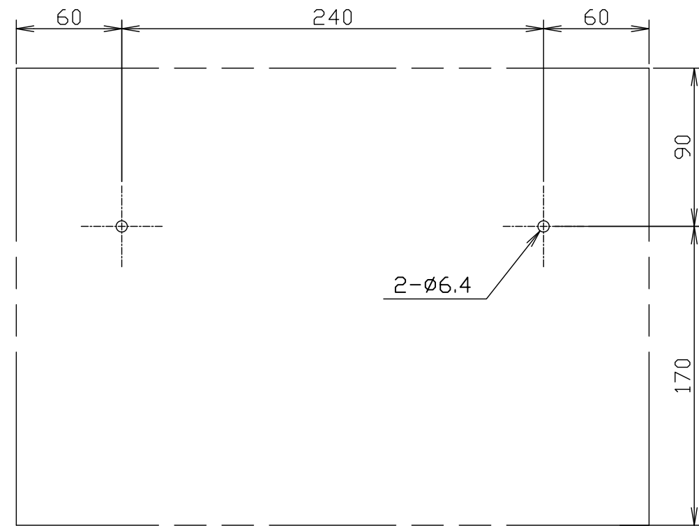
本体背板穴ピッチ (正面より見て)
