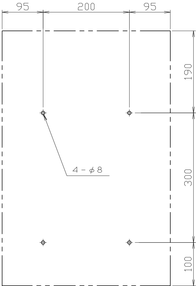
本体背板穴ピッチ
