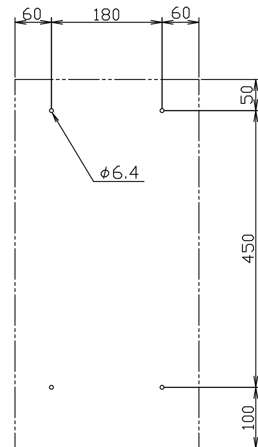
本体背板穴ピッチ(正面より見て)
