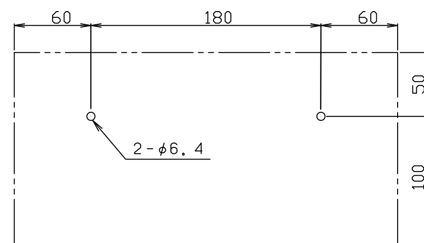
本体背板穴ピッチ（正面より見て）
