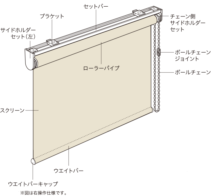
全体図
