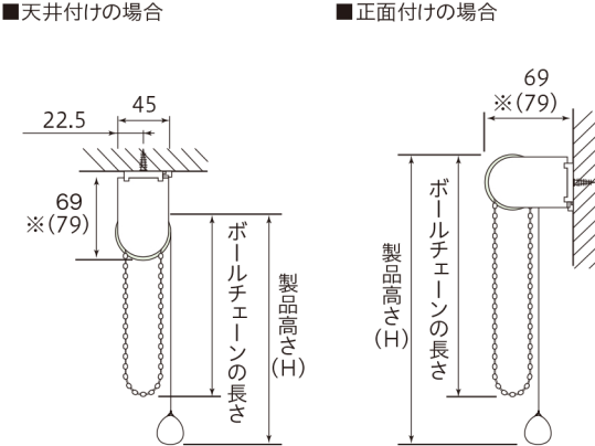
側面図 (mm)
