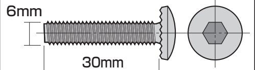
④ボルトB×4本 (M6×30)
