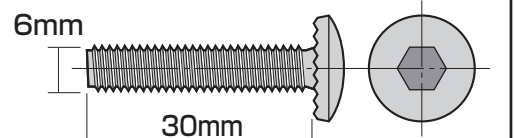
④ボルトB (M6×30)
