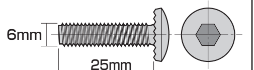
③ボルトA (M6×25)
