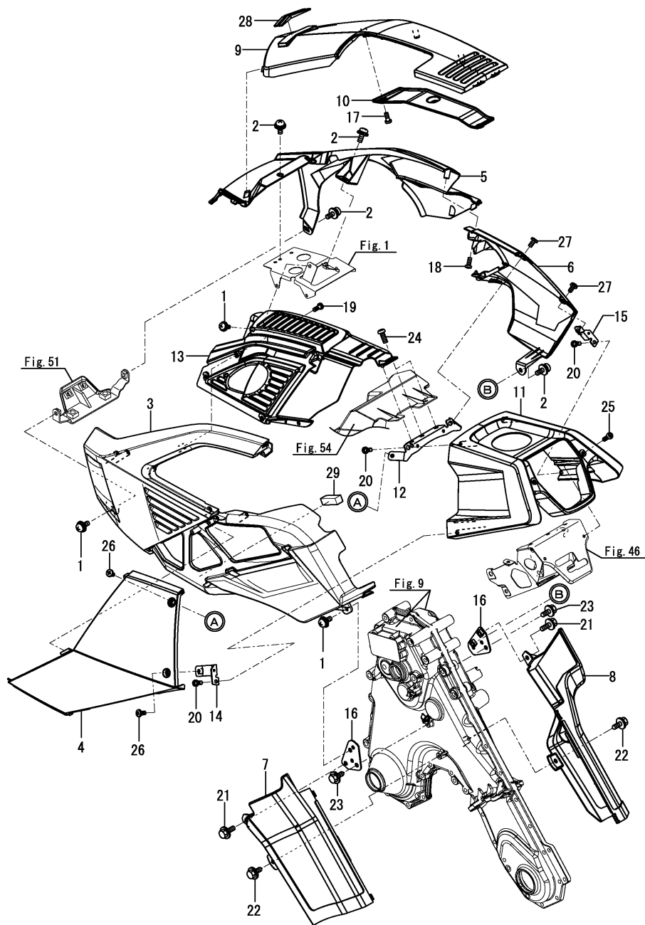
Fig.53. カバー
