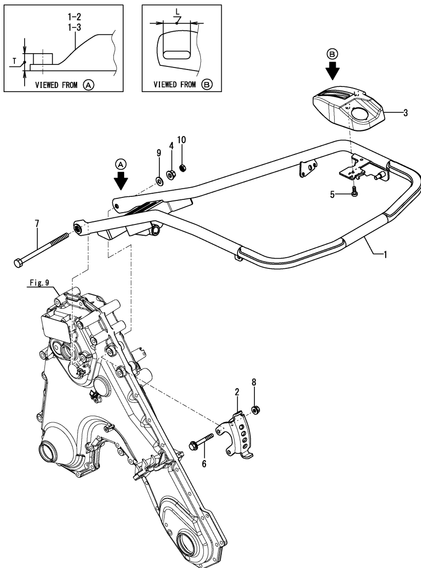
Fig.45. ハンドル
