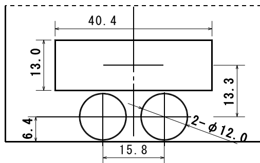
[7セグメントLED、スイッチ引き出し穴寸法]
