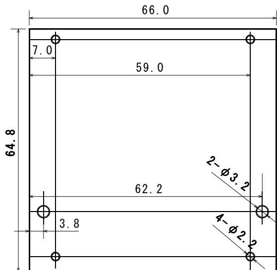
[基板取り付け穴寸法]
