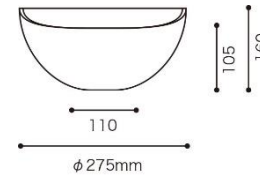
利休信楽 030-G275 濃紅(こきあか) φ275 × H160 × SH105 重量3.0Kg 税抜 ¥ 22.000-
