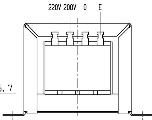
A 矢視図
