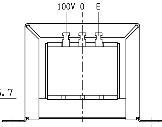
A 矢視図
