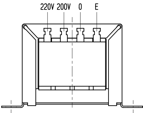
A 矢視図
