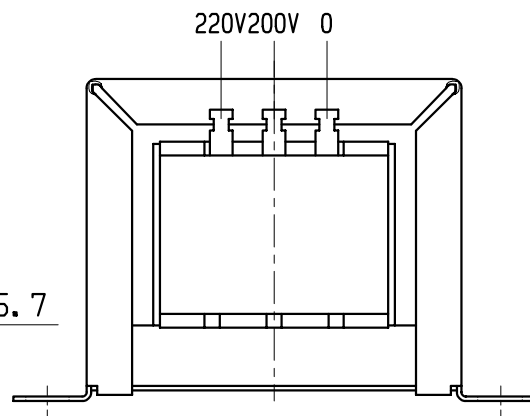
A 矢視図
