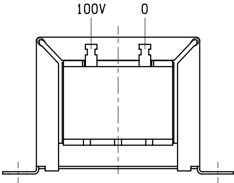
A 矢視図
