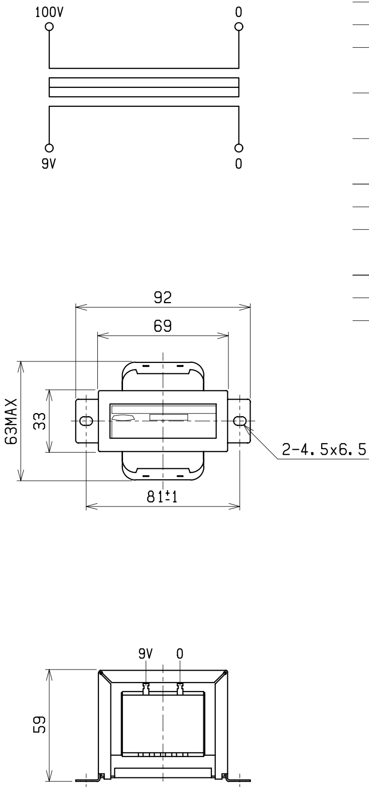
結 線 図
