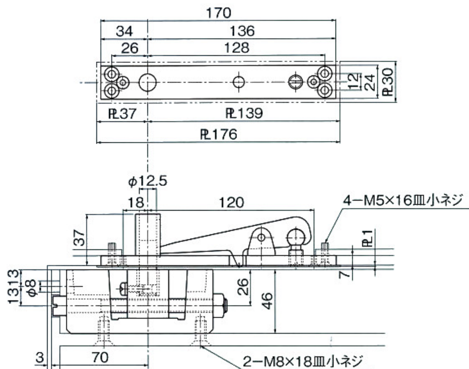
1 トップピボット(上枠側)
