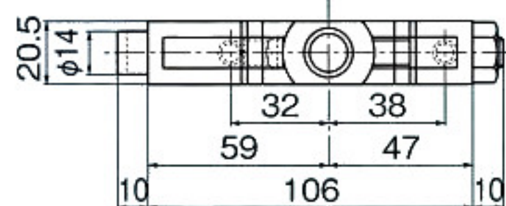
2 トップピボット(ドア側)
