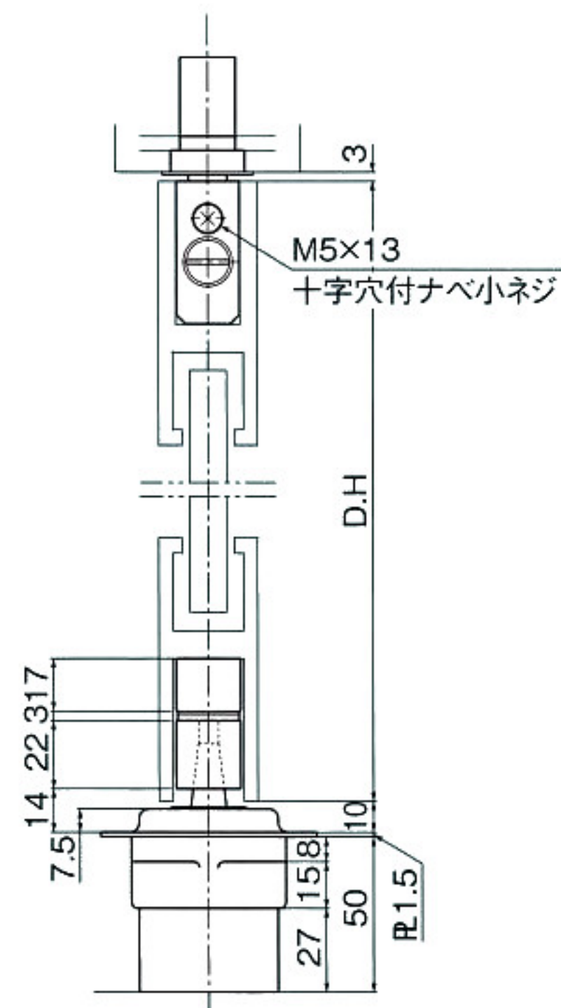
4 本体
