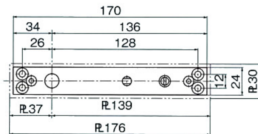
1 トップピボット(上枠側)
