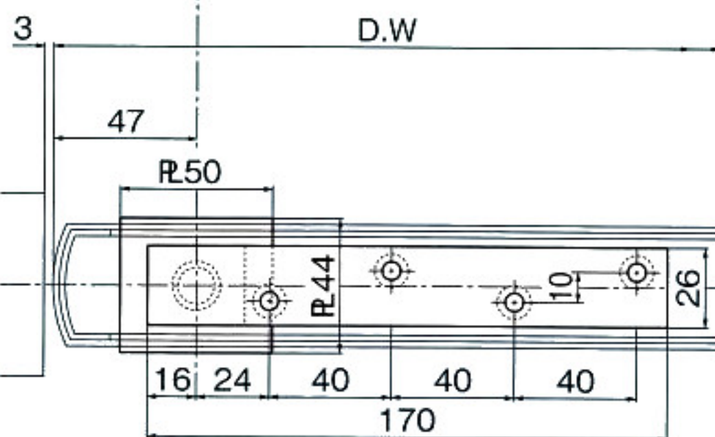
3 アーム(ドア側)
