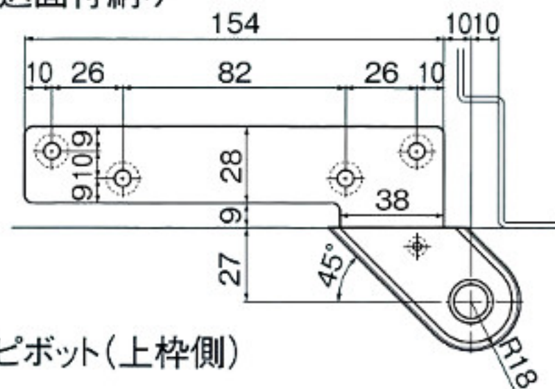
1 トップピボット(上枠側)掘込面付納り
