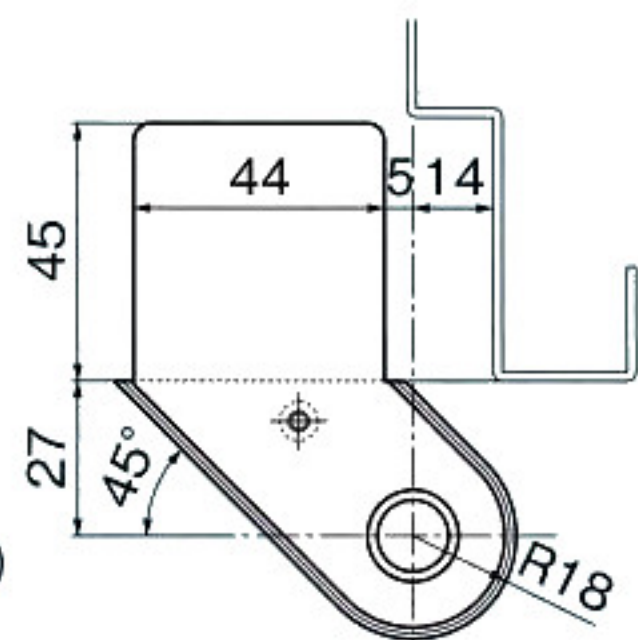
1 トップピボット(上枠側)
