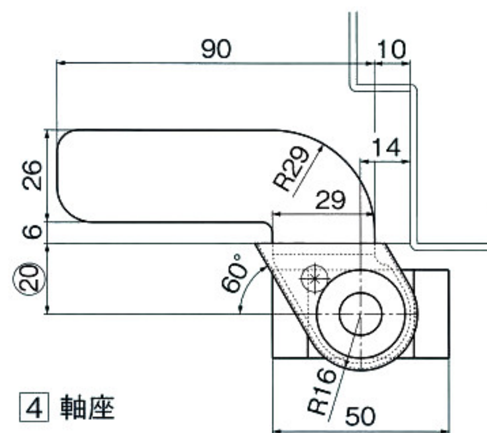
3 アーム(ドア側)
