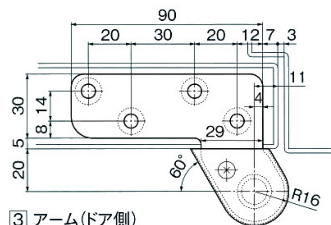
2 トップピボット(ドア側)
