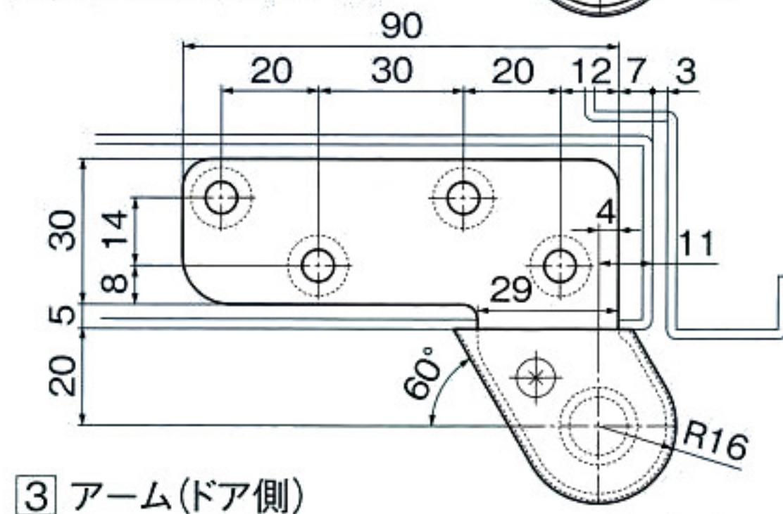
2 トップピボット(ドア側)
