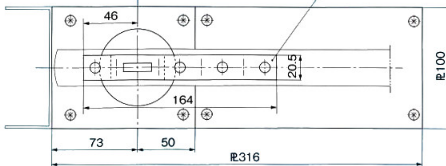
4 フロアヒンジ部品ナシ本体 (床側)
