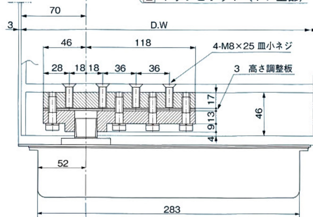
2 トップピボット (ドア上部)
