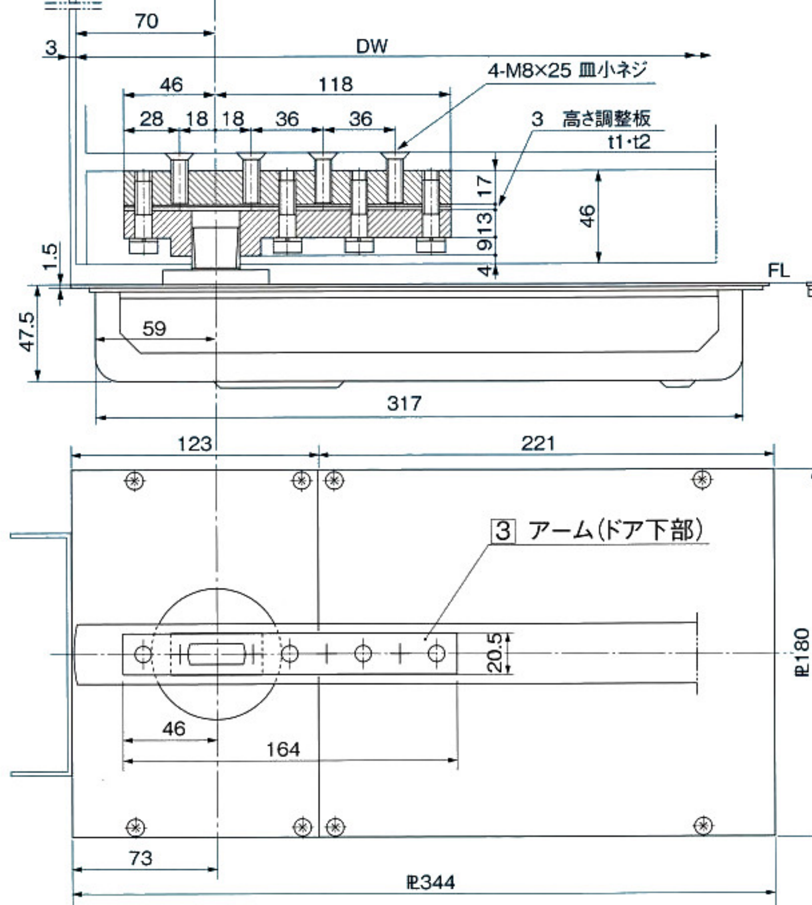
4 フロアヒンジ部品ナシ本体(床側)
