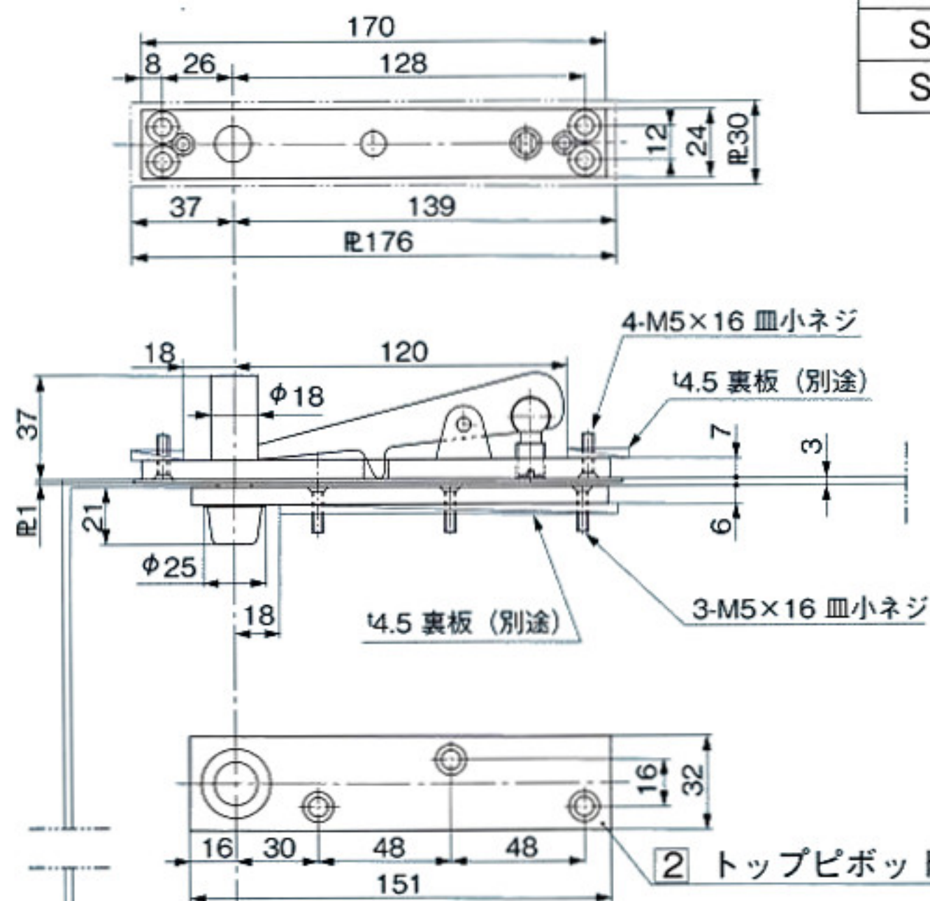
1 トップピボット (上枠側)
