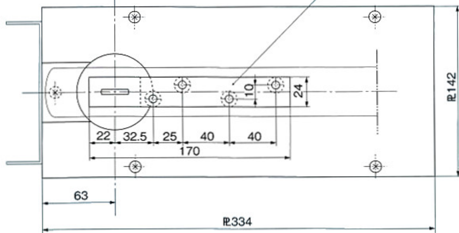
4 フロアヒンジ部品ナシ本体 (床側)
