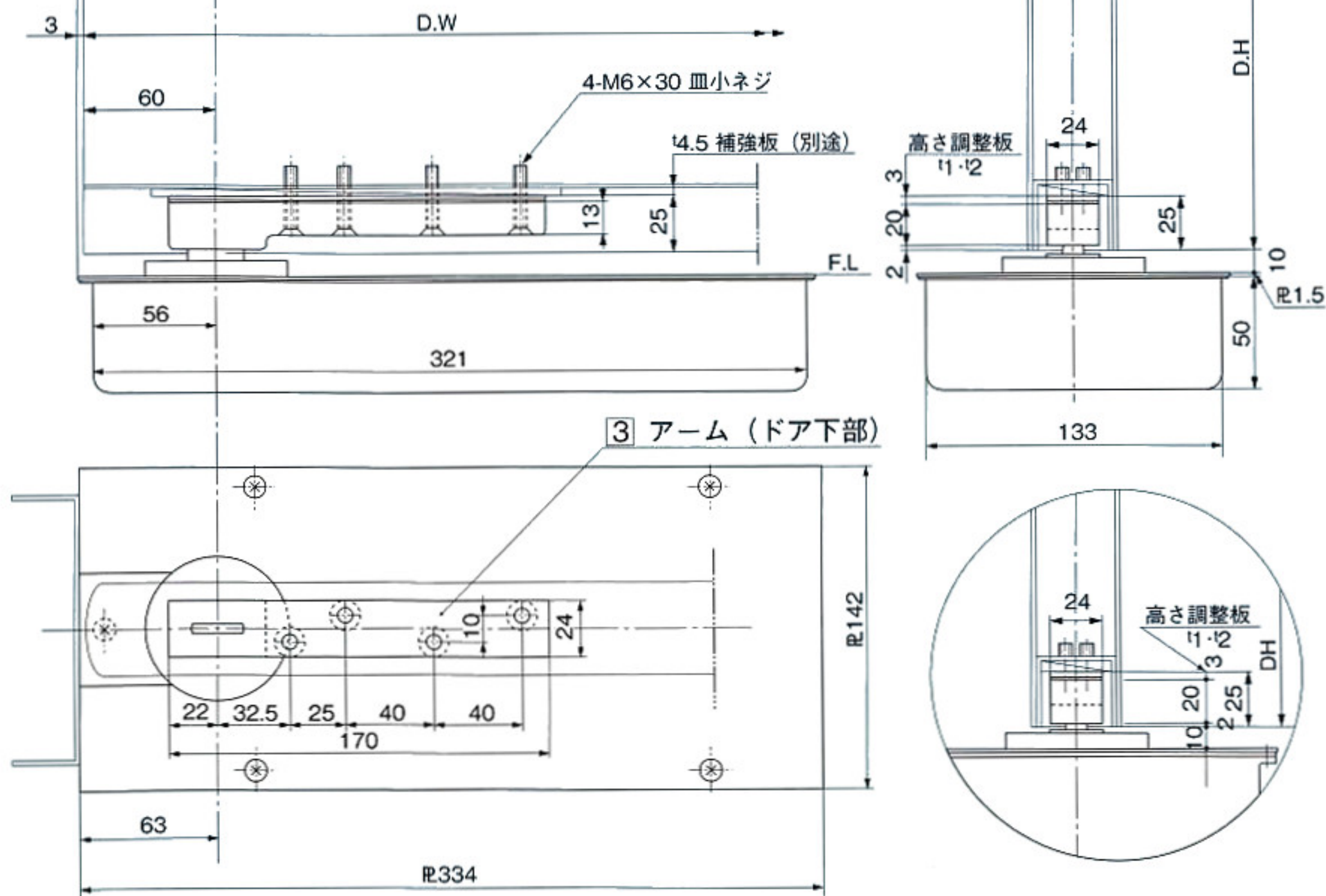
4 フロアヒンジ部品ナシ本体 (床側)
