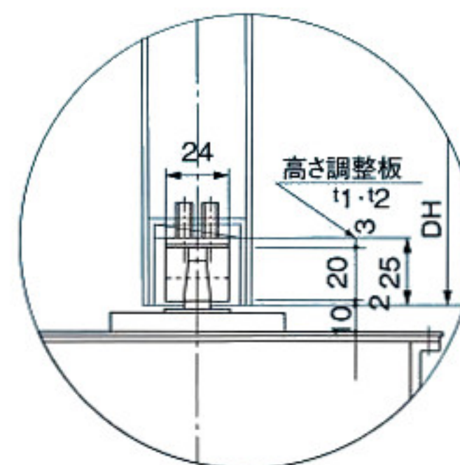
④ フロアヒンジ部品ナシ本体(床側)
