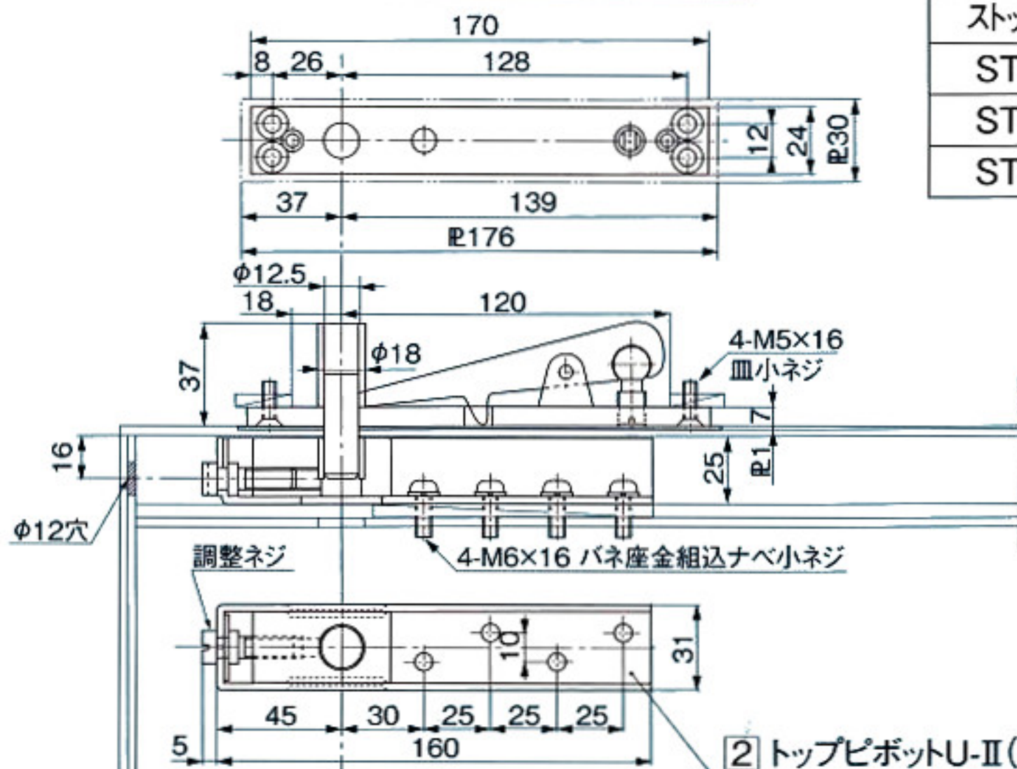
① トップピボット(上枠側)
