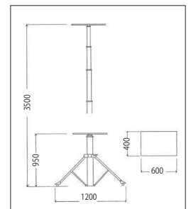
寸法図
