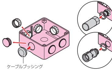
ケーブルブッシング
