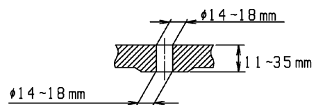
便座取付穴断面
