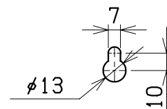
取付穴詳細図
